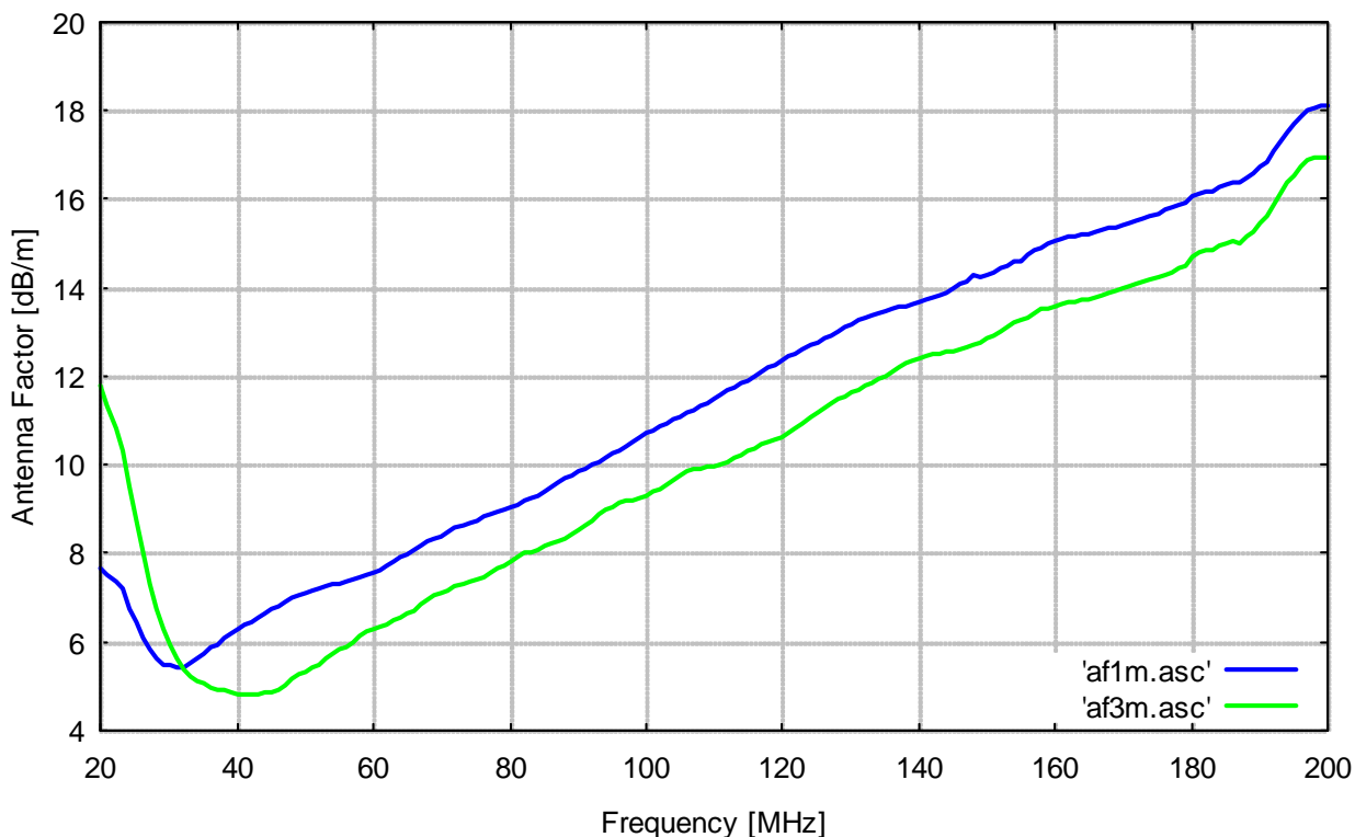
Antennen-Wandlungsmaß
